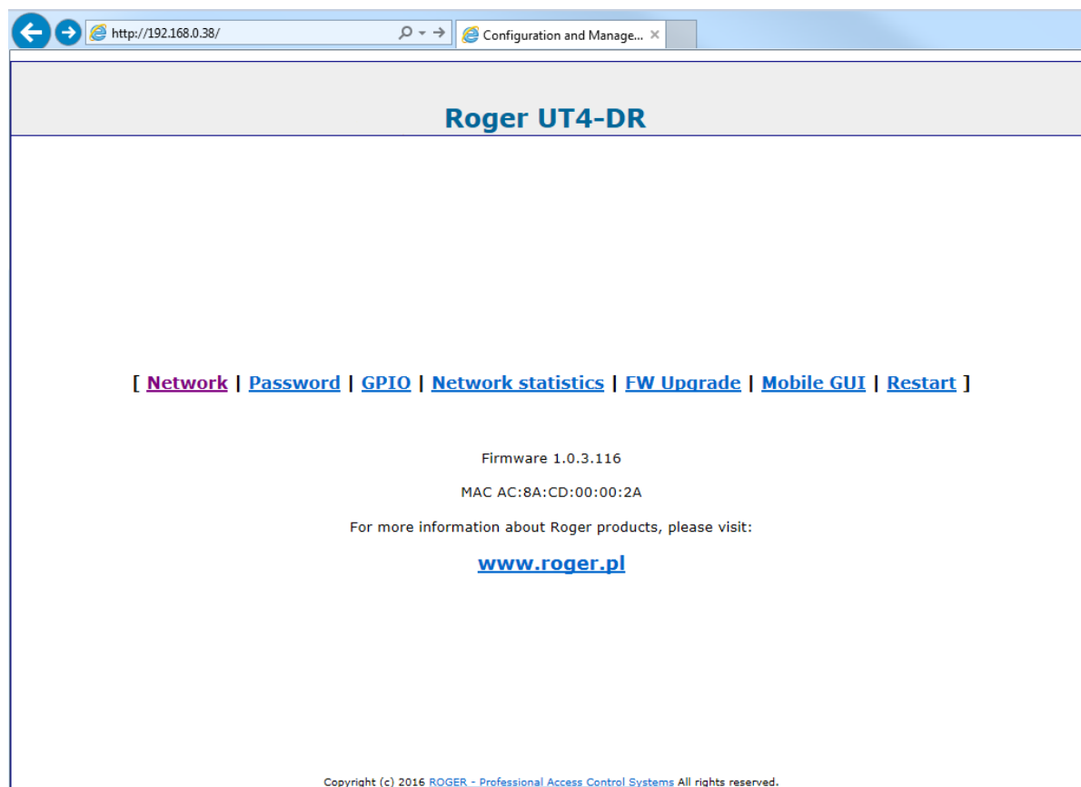
Rys. 4 Okno konfiguracyjne interfejsu UT-4DR w przeglądarce internetowej
